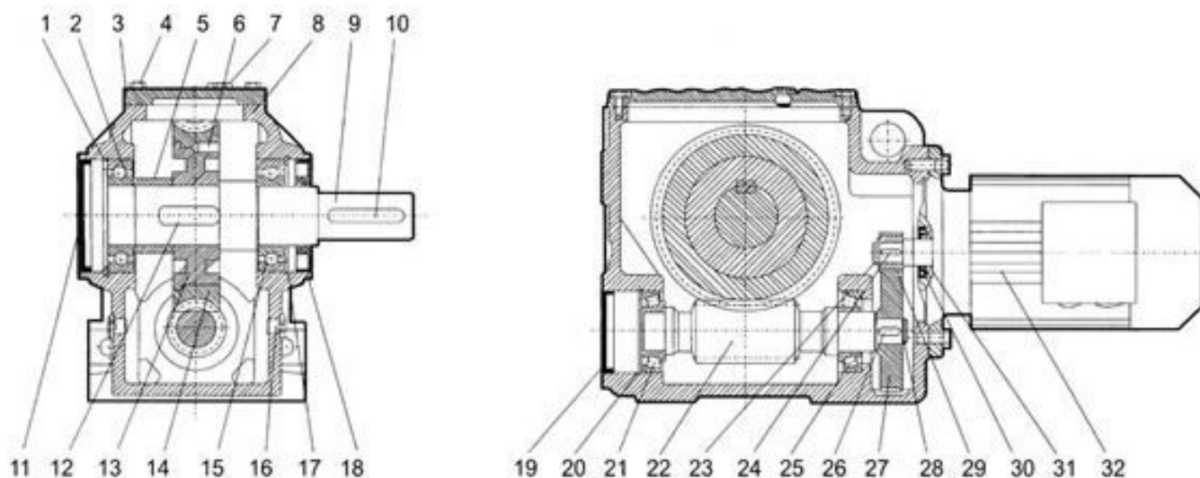
产品结构示意图
