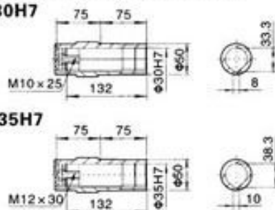
Φ30H7
